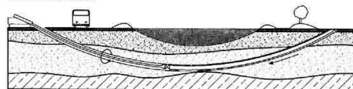
Rys.3) Przeciąganie rurociągu
