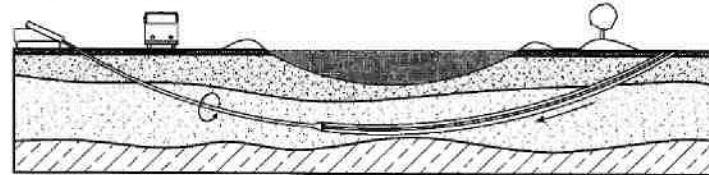
Rys.2) Poszerzanie otworu
